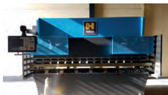
AV Presse plieuse HACO PPES 30150 Outillage rectifié - Vis à bille - Rétrofit complet Easybend - Moteurs neufs Tél : 03 20 10 30 40 Mail : commercial@haco.fr
