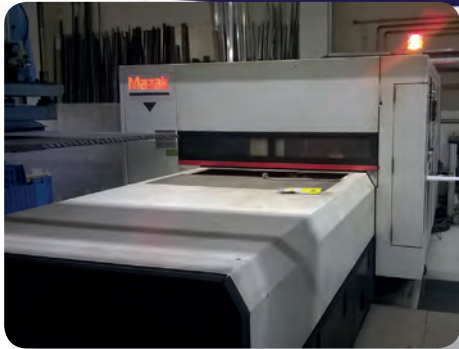
Laser MAZAK STX 48 4000 W Année 2012
