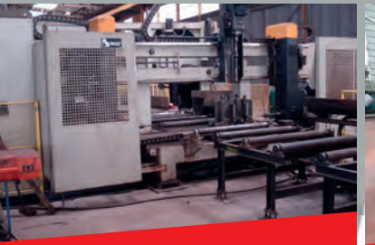
Centre de perçage et sciage FICEP 1203 DB Année 2000 Largeur 1250 mm - Longueur banc 18 m Capacité de perçage CM4
