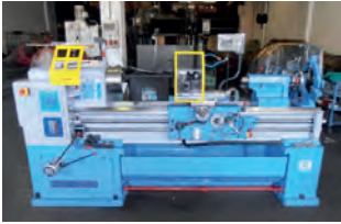
AV Tour parallèle CAZENEUVE - Type HB 575 x 1500 - Reconstitué - Distance entre pointe : 1500 mm - Hauteur de pointe : 250 mm - ø admis au dessus du banc : 575 mm - ø admis au dessus du chariot : 340 mm - Alésage broche : 52 - Conicité de la contre pointe : CM5 - Course maxi du chariot transversal : 400 mm - 18 vitesses de broche : 25 à 2000 tr/min - Puissance moteur de broche : 8,8 kW Dimensions machine : 2400 x 1180 x 1350 Protection mandrin - Tél : 06 07 68 86 74 Mail : lgmo95@orange.fr
