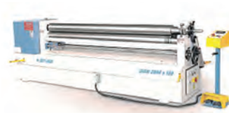
AV Encocheuse hydraulique à angle fixe ACCURL - Type AF 206 - Machine neuve Angle fixe : 90° - Réglage entre lames automatique - Dimension de la table : 650 x 650 mm - Longueur des lames : 200 mm - Coupe par minute : 40 mm Epaisseur max. acier : 6 mm - Epaisseur max. inox : 3 mm - Puissance moteur : 5,5 kw - Encombrement : 1500 x 1400 x 1580 mm - Poids : 1950 kg
