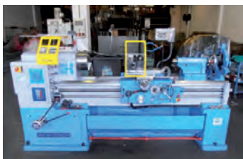
AV Tour parallèle CAZENEUVE - Type HB 575 x 1500 - Reconstituit - Distance entre pointe : 1500 mm - Hauteur de pointe : 250 mm - ø admis au dessus du banc : 575 mm - ø admis au dessus du chariot : 340 mm - Alésage broche : 52 - Conicité de la contre pointe : CM5 - Course maxi du chariot transversal : 400 mm - 18 vitesses de broche : 25 à 2000 tr/min Puissance moteur de broche : 8,8 kw Dimensions machine : 2400 x 1180 x 1350 Protection mandrin Tél : 06 07 68 86 74 Mail : lgmo95@orange.fr
