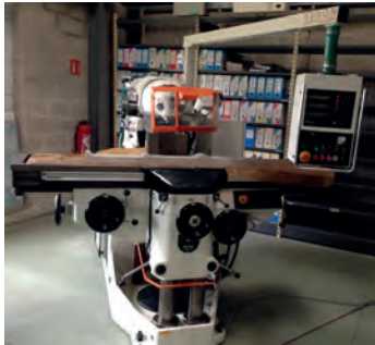
AV Fraiseuse conventionnelle HURON Type MU6 - Table : 2000 x 460 mm Courses : 1500 x 700 x 500 mm Commandes sur pendentif - Machine reconstruite - Tél : 05 61 78 85 85
