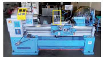
AV Tour parallèle CAZENEUVE - Type HB 575 x 1500 - Reconstitué - Distance entre pointe : 1500 mm - Hauteur de pointe : 250 mm - ø admis au dessus du banc : 575 mm - ø admis au dessus du chariot : 340 mm - Alésage broche : 52 - Conicité de la contre pointe : CM5 - Course maxi du chariot transversal : 400 mm - 18 vitesses de broche : 25 à 2000 tr/min Puissance moteur de broche : 8,8 kw Dimensions machine : 2400 x 1180 x 1350 Protection mandrin Tél : 06 07 68 86 74 Mail : lgmo95@orange.fr
