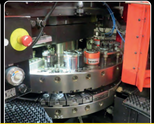
Poinçonneuse AMADA Electrique AE 255 NT avec Chargeur LKI MP250 (état neuf 2011) - Nombreux outillages avec placard
