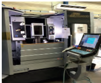
AV Erosion SODICK ALC 400G - Année 2017 - Courses : 400 x 300 x 250 mm Poids maxi pièce : 500 kgs - U/V axis : 150 x 150 mm - Dimensions du bac : 850 x 610 mm - Enflage automatique Immersion - Groupe froid - Nombre d'heures : 5 600 h - Tél : 04 74 73 80 48 Mail : emoventeachat@outlook.fr
