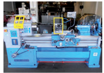
AV Tour parallèle CAZENEUVE - Type HB 575 x 1500 - Reconstitué - Distance entre pointe : 1500 mm - Hauteur de pointe : 250 mm - ø admis au-dessus du banc : 575 mm - ø admis au-dessus du chariot : 340 mm - Alésage broche : 52 - Conicité de la contre pointe : CM5 - Course maxi du chariot transversal : 400 mm - 18 vitesses de broche : 25 à 2000 tr/min - Puissance moteur de broche : 8,8 kw - Dimensions machine : 2400 x 1180 x 1350 - Protection mandrin Tél : 06 07 68 86 74 Mail : lgmo95@orange.fr
