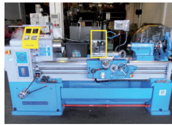
AV Tour parallèle CAZENEUVE - Type HB 575 x 1500 - Reconstitué - Distance entre pointe : 1500 mm - Hauteur de pointe : 250 mm - \phi admis au-dessus du banc : 575 mm - \phi admis au-dessus du chariot : 340 mm - Alésage broche : 52 - Conicité de la contre pointe : CM5 Course maxi du chariot transversal : 400 mm - 18 vitesses de broche : 25 à 2000 tr/min - Puissance moteur de broche : 8,8 kw - Dimensions machine : 2400 x 1180 x 1350 - Protection mandrin Tél : 06 07 68 86 74 Mail : lgmo95@orange.fr
