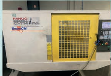
Centre d'usinage FANUC ROBODRILL T14 iFLB Occasion Courses 700 x 400 x 330 mm Diviseur FANUC
