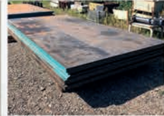
Marbre lisse en fonte 3910 x 2000 x épaisseur 350 mm Poids env 7 T Fournis avec 6 pieds de nivellement (2 marbres identiques disponibles) + autres dimensions disponibles
