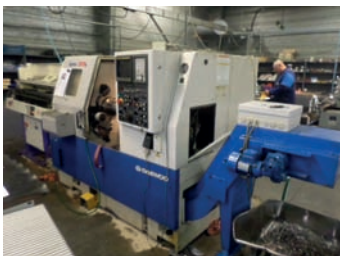
AV Tour CNC DAEWOO Lynx 200 LC De 2001 - CNC Fanuc 21T - Embarreur Tél : 03 88 72 02 47
