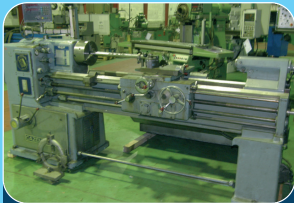
Tour CAZENEUVE HB 500 x I 500 Diam sur banc : 500 mm - EP : I 500 Visu 2 axes + tourelle MULTIFIX + Lunette
