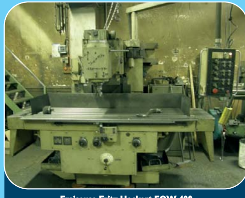
Fraiseuse Fritz Heckert FQW 400 Table : 2 000 x 400 mm Courses : X 1 400, Y 560, Z 460 Broche : 15 kw
