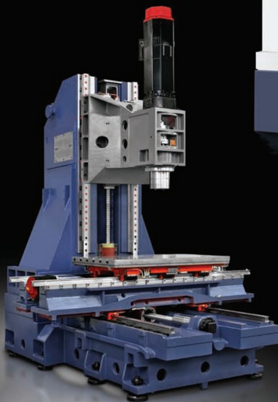
Guidage de l'axe X par 6 patins largement dimensionnés
