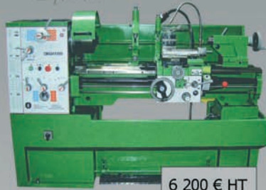
Tour conventionnel de précision REF. S-M6241x1000
