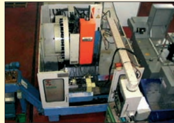
Centre d'usinage vertical MAZAK V414 Mazatrol M32 Diviseur 4 ème axe Nikken Petit prix
