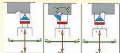
Diamanteur numérique 3 axes
