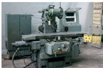
Fraiseuse ERNAULT SOMUA Type Z3C 1 000 x 320 x 470 mm 10 000€ - 3 000€
