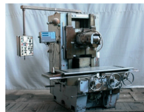
Fraiseuse VERNIER Type FV750 1 250 x 500 x 800 mm 5 000€ - 3 000€
