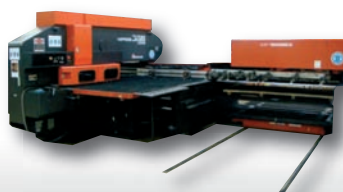
Poinçonneuse CNC AMADA VIPROS 358 KING 30 T - 1 270 x 4 000 mm avec repos. CN Fanuc - Tourelle 58 outils 4 auto index Chargeur / déchargeur MP 1225EX 1998
