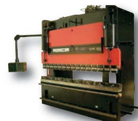
Presse plieuse AMADA PROMECAM - STPC 200 T x 3 000 mm CNC 5 axes
