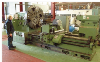
Tour GURUTZPE - B 2000 ø usinable 1600 mm - Entre pointe 2300 mm
