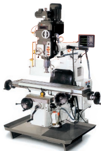
Fraisuse à tourelle FTV 5-SP Table : 1372 x 280 mm Rainures en "T" : 3 x 16 x 63 mm Courses : 800 x 345 x 400 mm
