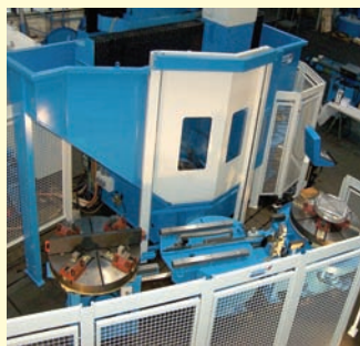
BERTHIEZ LVM 125 P (1987/2007), palettisé, Ø 1.250 / 1.600 mm, axe C, outils tournants, CN SIEMENS 840 D.
