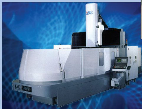
Centre d'usinage KAO MING X 1500 à 8000 - Y 1000 à 3450 - Changeur d'outils
